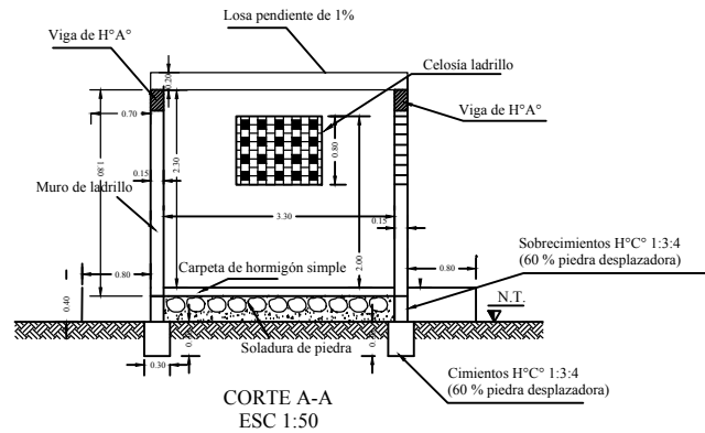
DETALLE CONSTRUCCION DE CASETA DE BOMBEO
